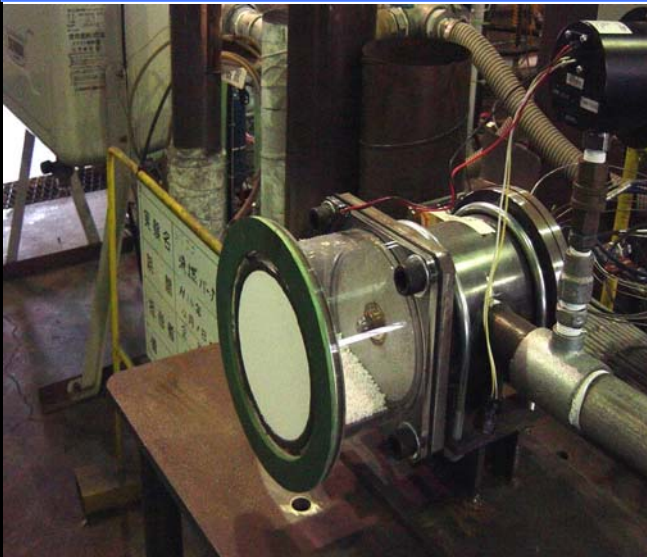
スプレーノズル整流実験用バーナ
