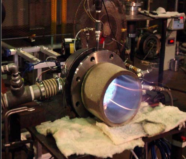
油焚きボイラ用気泡分散予混合燃焼バーナ
