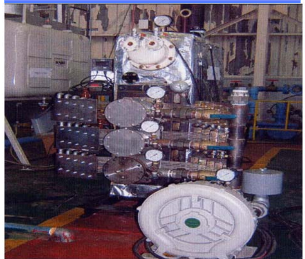
気泡分散バーナ搭載プロトタイプボイラ
